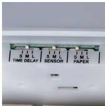
Sensor (Einstellmöglichkeiten)
